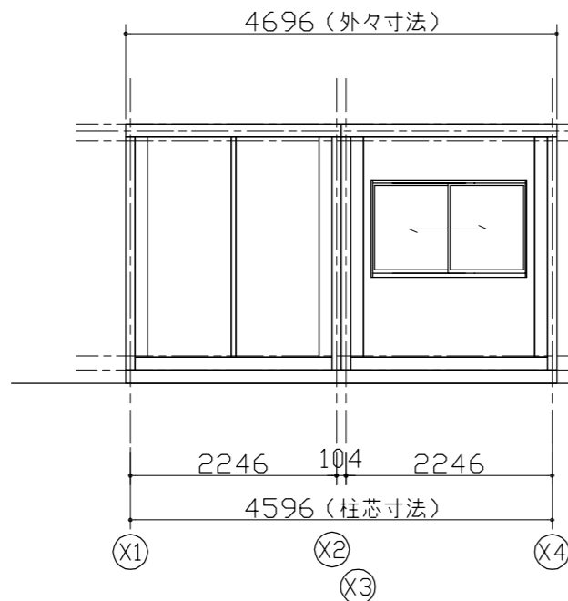
(Y1) 通り立面図
